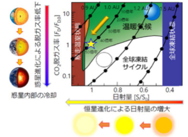
図4 ハビタブルゾーンにおいて地球の軌道要素を変えた場合の惑星の気候進化。地球の熱進化の結果、二酸化炭素の脱ガス率が低下し、一方で恒星進化の結果、太陽光度は増加するため、左下りの進化トラックとなる (Kadoya and Tajika, 2015).
