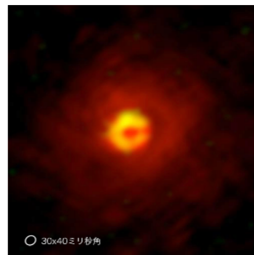
図2 ALMA望遠鏡で観測したうみへび座W星のガス分布。明るい部分がAlO分子、暗い部分が29SiOの分布。AlO分子が恒星近傍で塵を形成している(ALMA(ESO/NAOJ/NRAO), Takigawa et al. 2017)。
