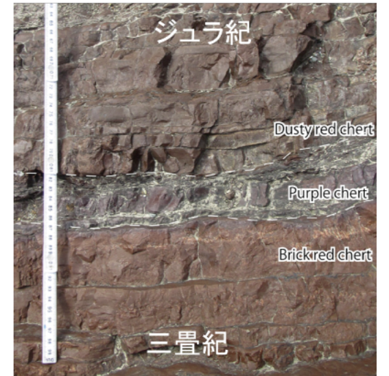
図4 層状チャートの堆積リズム（縞々）に刻まれた天文学的周期 (Ikeda and Tada, 2020)
