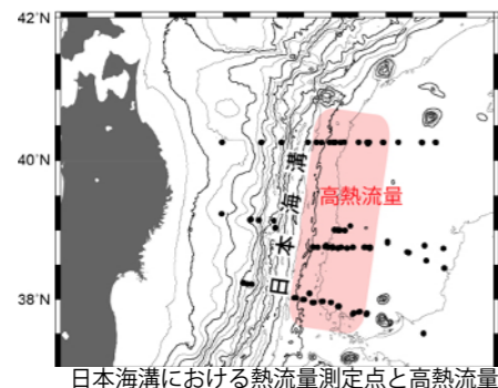
日本海溝における熱流量測定点と高熱流量
