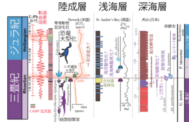
図2 三疊紀/ジュラ紀境界における陸-浅海-深海の層序対比 (Ikeda et al., 2015).
