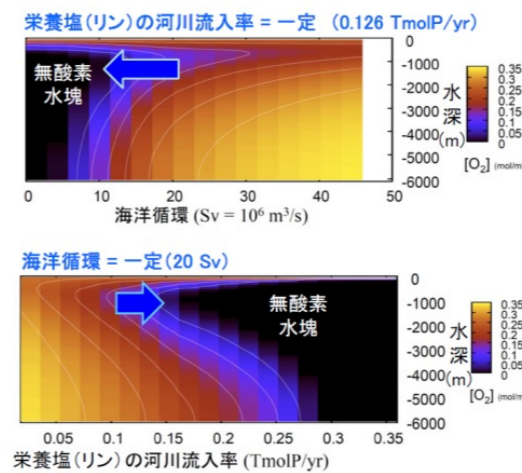
図3 海洋生物化学循環モデルを用いた海洋無酸素イベントの数値シミュレーション。海洋循環が停滞する栄養塩の河川流入率増加によって生物生産が増加すると無酸素水塊が発達する (Ozaki et al., 2011).
