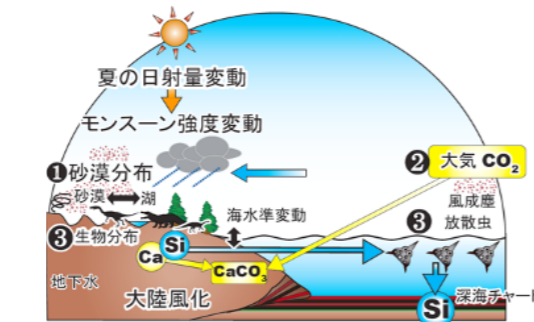
図1：地球軌道変化が地球環境に与える概念図 (Ikeda et al., 2017).
