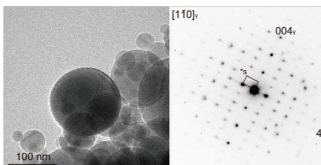
図1 透過型電子顕微鏡で撮影した誘導熱プラズマ装置で合成した星周塵模擬粒子(左)。中央のAl 2 O 3 粒子はこれまでに報告されたことのない結晶構造をもつ(右)
