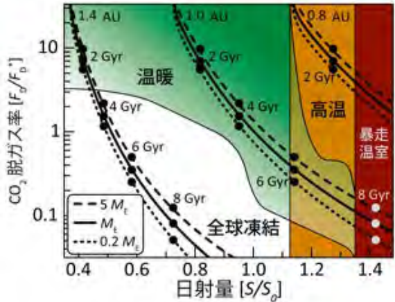
図4 ハビタブルゾーンにおいて地球の軌道要素を変えた場合の惑星の気候進化。地球の熱進化の結果、二酸化炭素の脱ガス率が低下し、一方で恒星進化の結果、太陽光度は増加するため、右下がりの進化トラックとなる (Kadoya and Tajika, 2015)。
