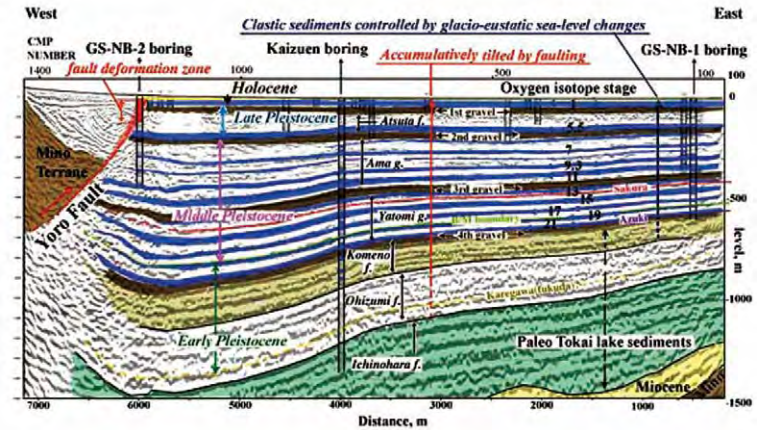
濃尾平野の地下構造（地質調査所速報による）。海成層と陸成層の互層が，みごとに発達している。図の左端には低角逆断層の養老断層が認められる。
