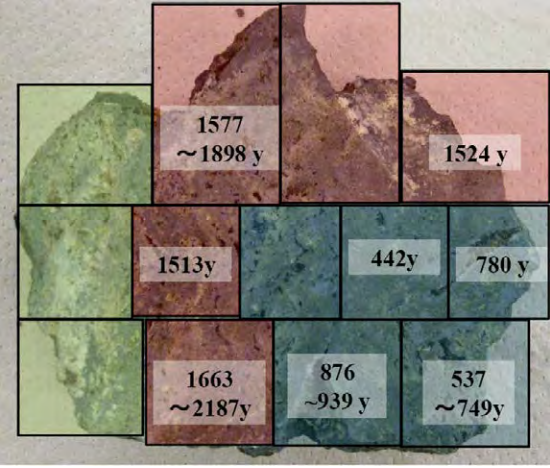
南マリアナトラフの熱水活動域で採取された硫化鉱物のクラスト（左）とその断面の U-Th 放射非平衡年代。20cm の断面が 1000 年以上の時間をかけて成長したことが分かる。
