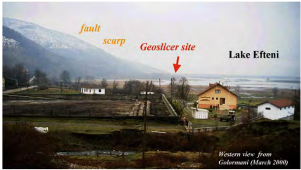
トルコ，北アナトリア断層系 1999 年 Duzce 地震断層。1999 年 8 月の Izmit 地震発生から約 3 ヶ月後の 11 月に Duzce 地震が発生した。Efteni 湖の湖畔には縦ずれ 2.6m，右横ずれ 2.7m の地表地震断層が出現した。
