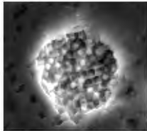
貧酸素環境を示す硫化鉱物
